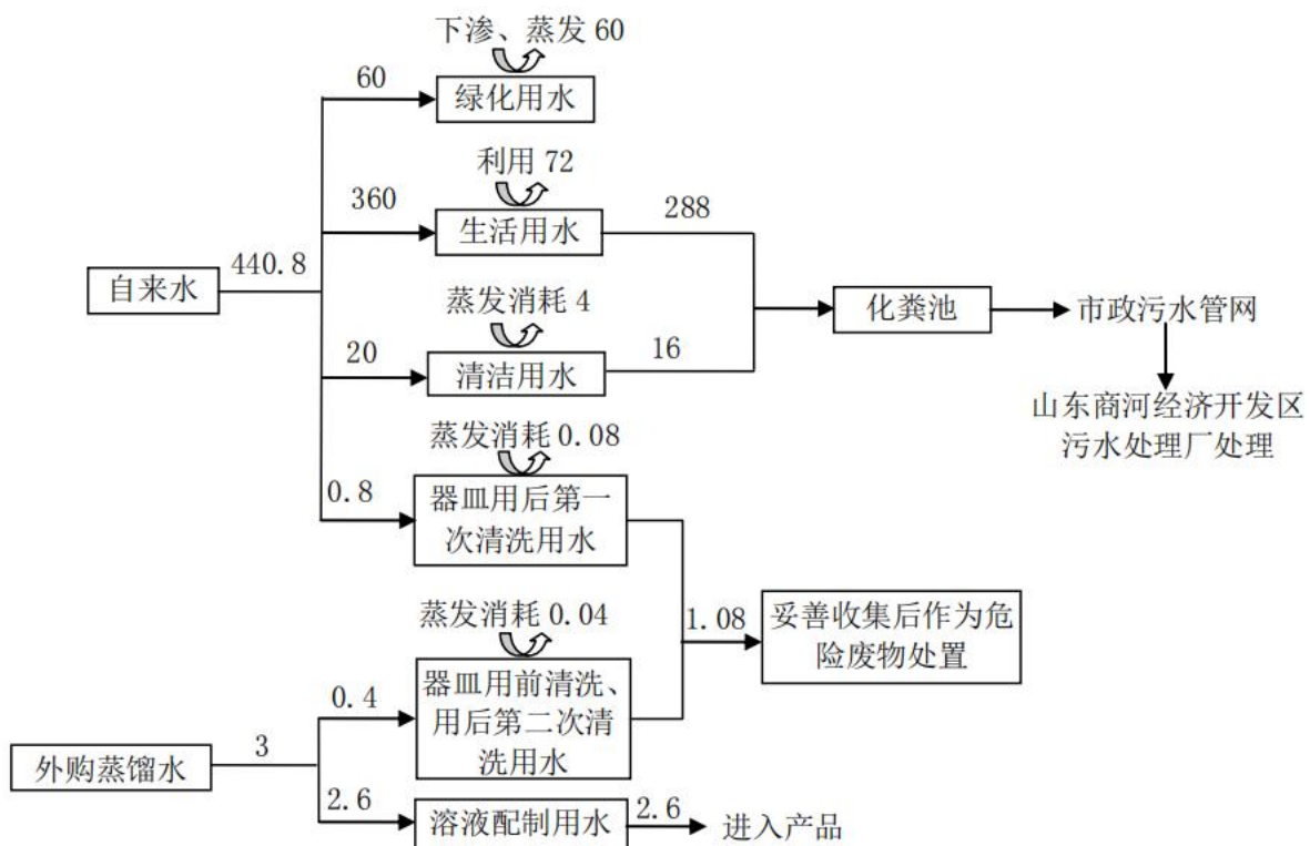
图3-3 废水处理工艺流程图
