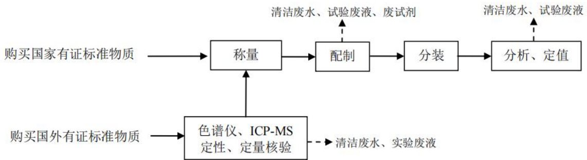
图2-3 工艺流程及排污节点图
