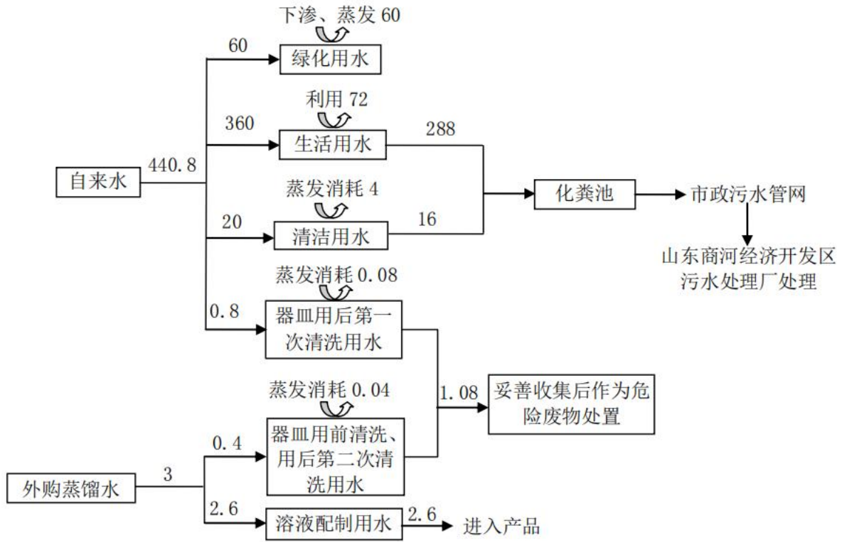
图2-1 项目水平衡图 (m³/a)
